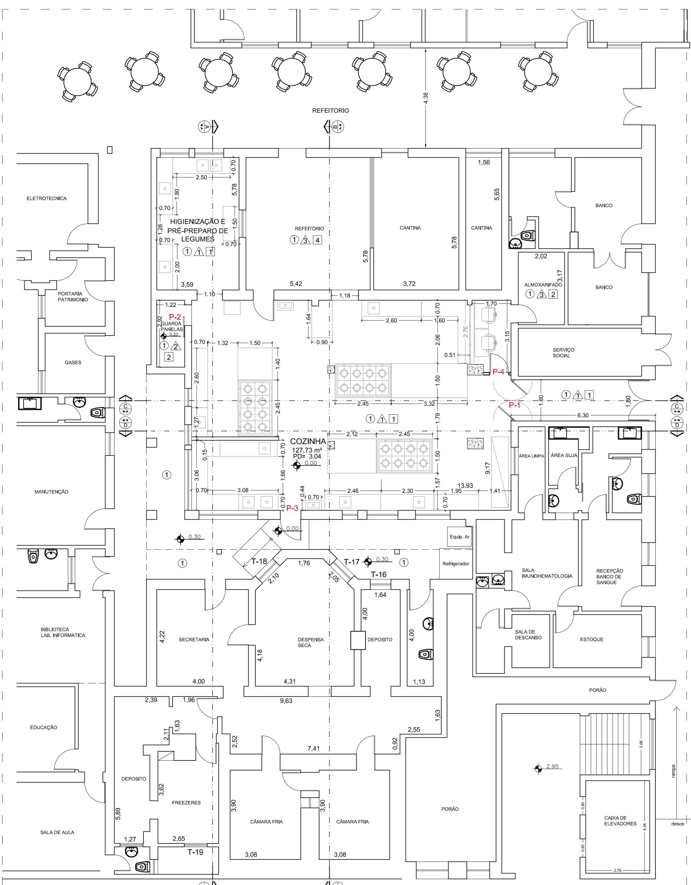
PLANTA BAIXA PAV. TÉRREO - (A EXECUTAR) (PROPOSTA 02) escala 1:100
